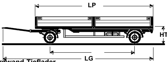
Bordwand-Tieflader
